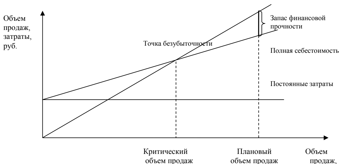
Рис. 3. График безубыточности
