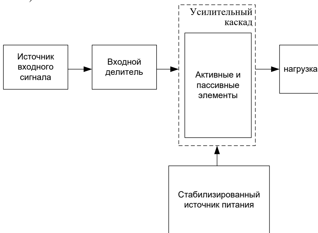
Рисунок 2.1 – Структурная схема усилительного каскада
