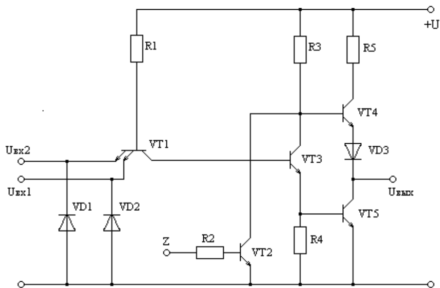
Рисунок 2.4 – Принципиальная электрическая схема базового элемента ТТЛ логики
