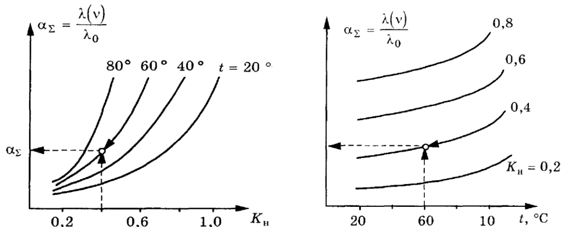
Рисунок 2.5 – Номограммы для определения произведения поправочных коэффициентов в случае учета двух факторов - коэффициента нагрузки и температуры
