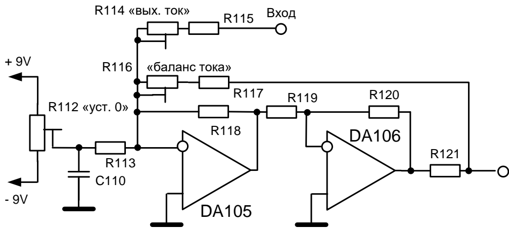
Рисунок 2.3 – Электрическая схема выходного преобразователя напряжение-ток
