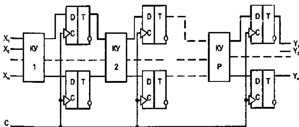
Рисунок 2.2 – Функциональная схема универсального регистра
