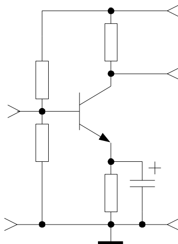
Рисунок 2.6 – Схема для примерного расчета показателей надежности
